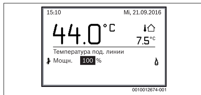
Рис. 29 Активен режим "трубочист"
