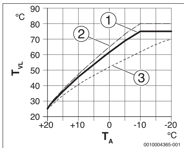
Рис. 37 Настройка отопительной кривой для радиаторов Угол наклона определяется расчётной температурой T_{VL} и минимальной наружной температурой T_{A,min}
