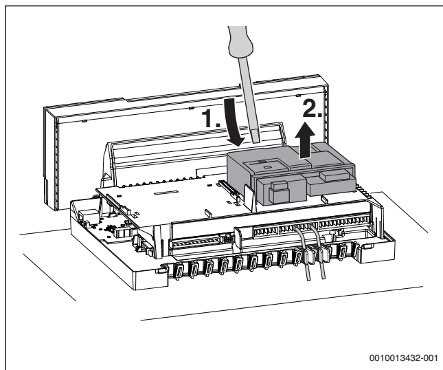
Рис. 16 Снятие функционального модуля
