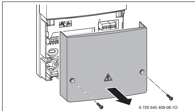
Рис. 7 Откройте корпус
