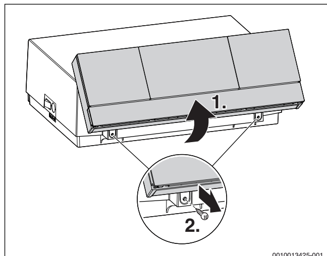
Рис. 3 Отверните винты
