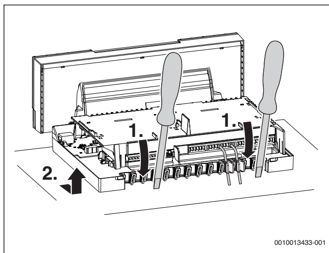
Рис. 17 Снятие системы управления с котла
