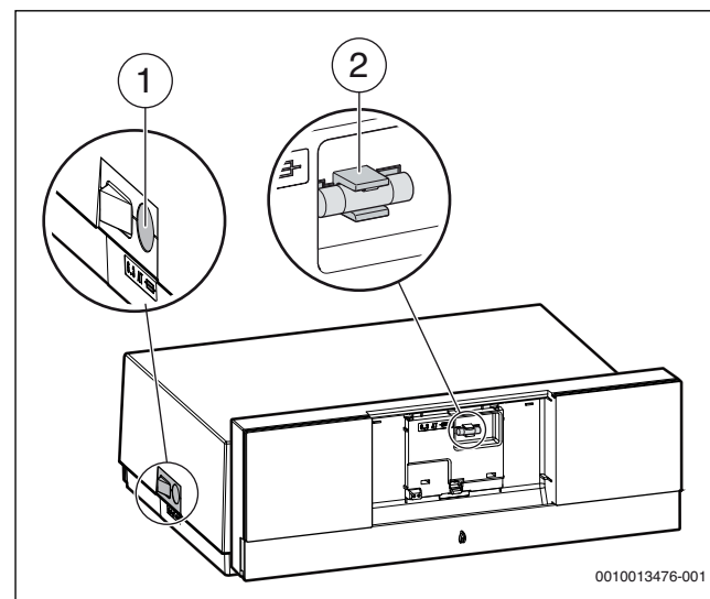
Рис. 41 Замена предохранителя
