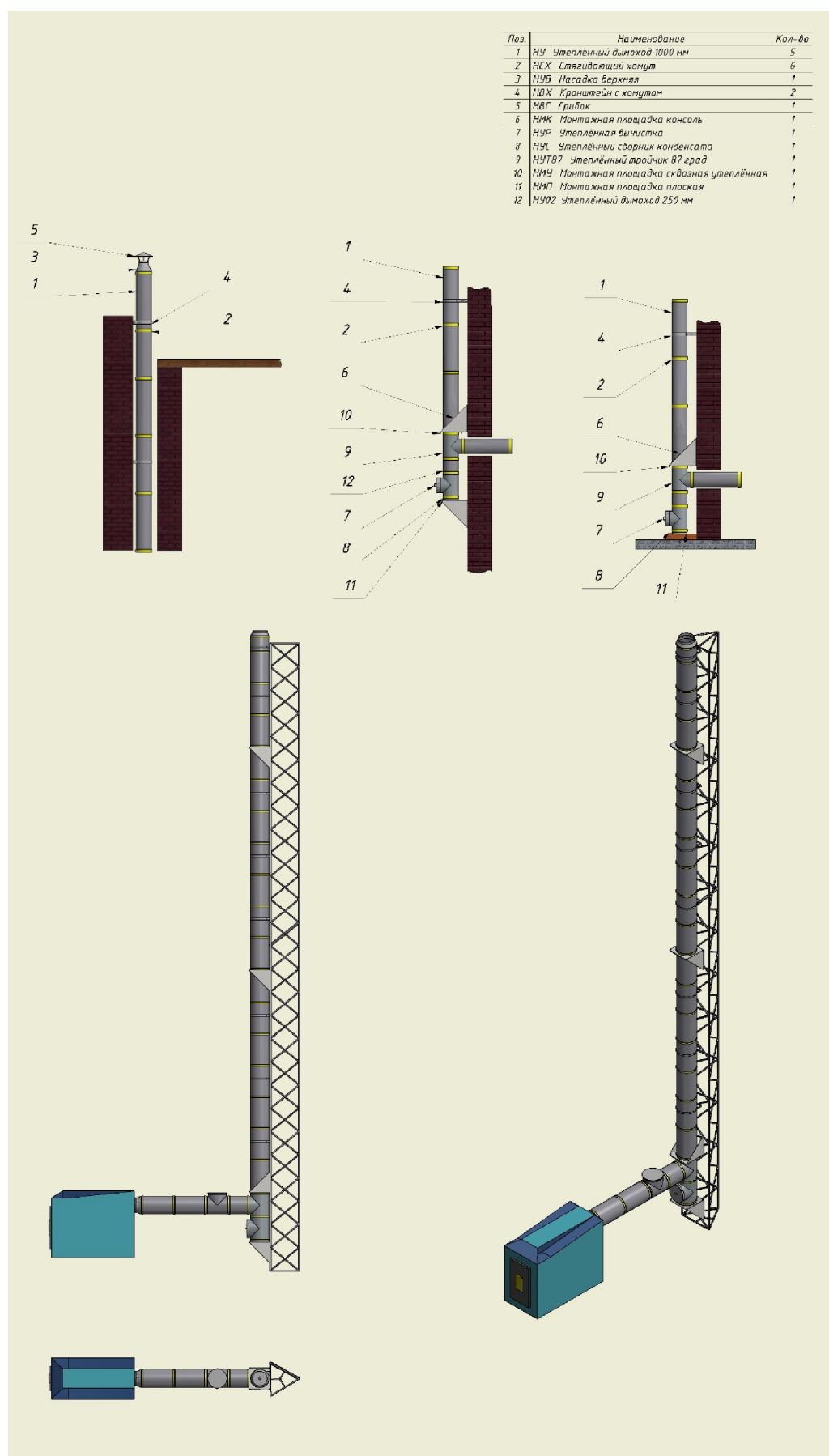
Рис.4 Пример двустенной системы дымоходов «Балтвент»
