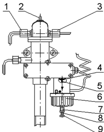
Рисунок 2. Блок автоматики
