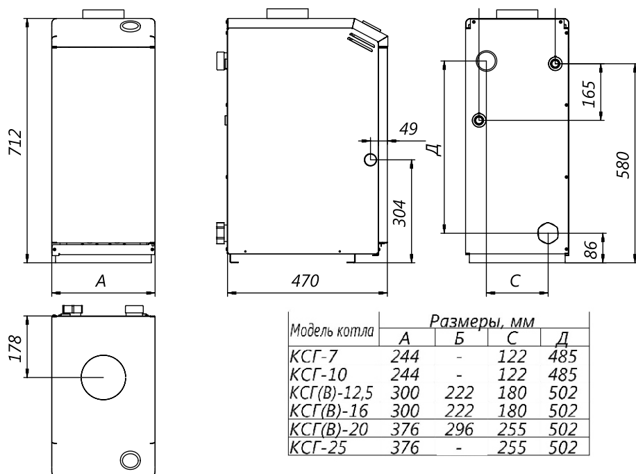
Рисунок 1 - Общий вид, габаритные и присоединительные размеры котлов модели «КСГ(В)»
