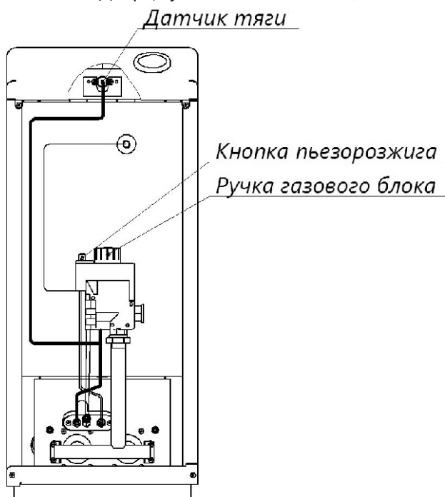
Рисунок 4 - Особенности котла с газовым блоком 630 EUROSIT
