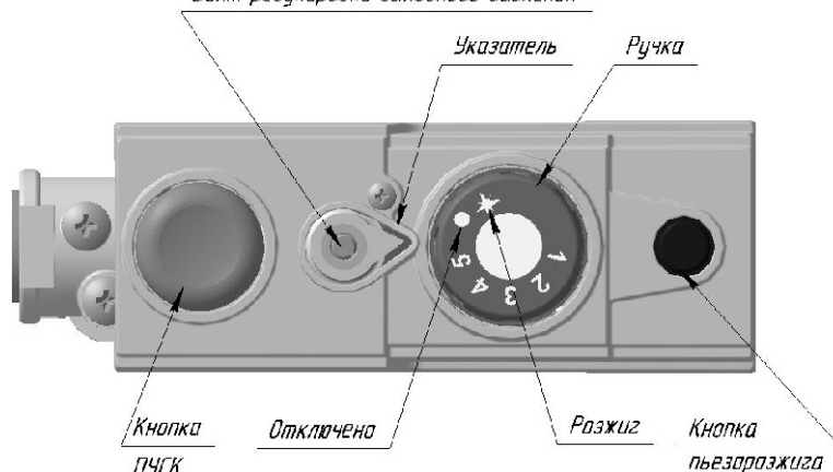
Рисунок 3. Элементы управления на газовом блоке автоматики САБК-АТ
