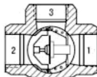
Позиции штуцеров автоматического трехходового клапана:
