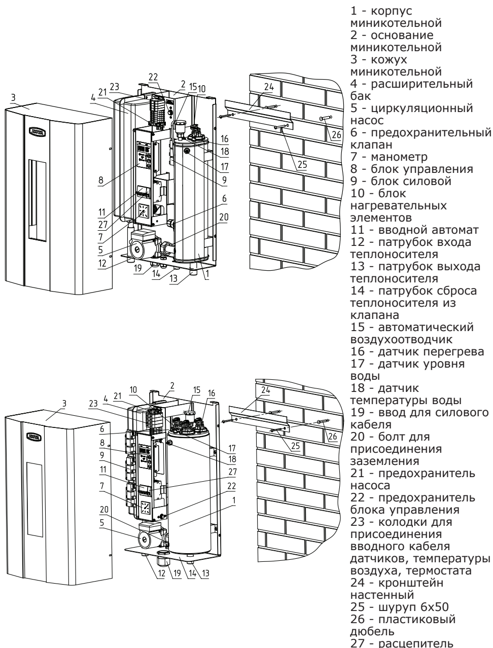
Рис. 1 Конструкция миникотельной и способ её крепления к стене ZOTA «МК» 3-15 / ZOTA «МК» 18-36
