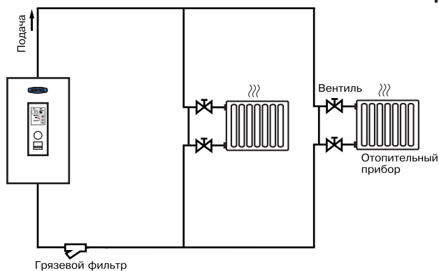
Рис. 9 Упрощенная схема подключения миникотельной в отопительную систему
