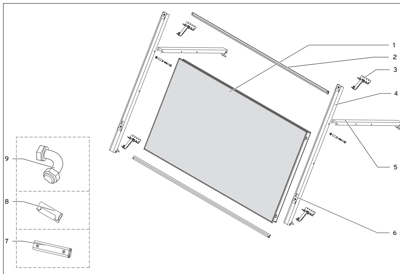
Рис. 5.4 Монтажный комплект VFK 135/2 D
