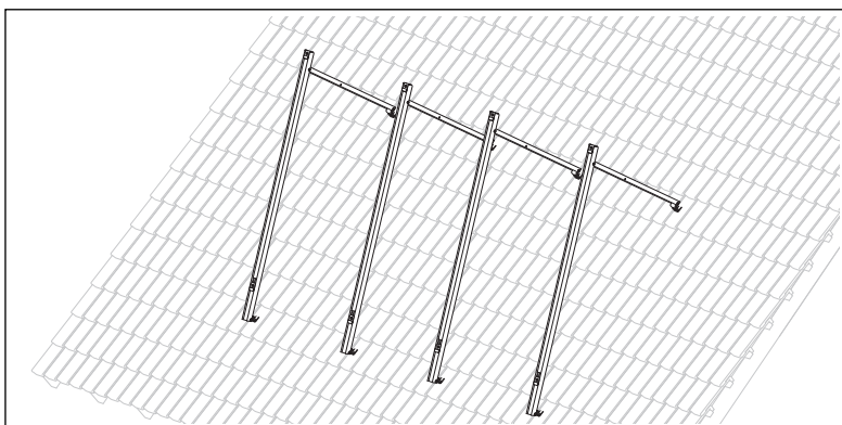
Рис. 5.15 Крепление каркасов
