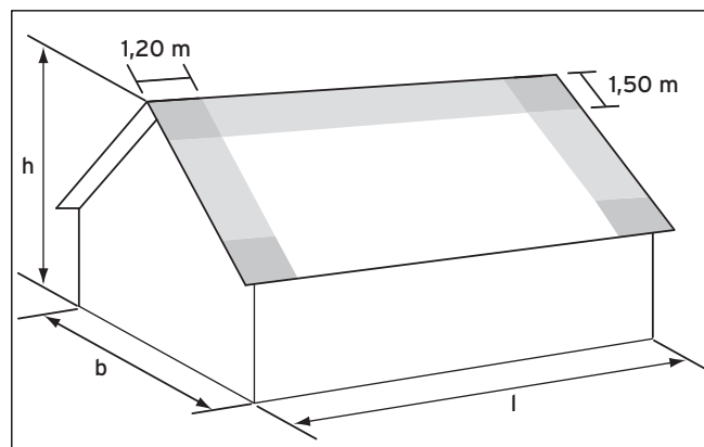
Рис. 5.5 Пример дома на одну семью, 12 м x 15 м x 8 м (ширина b /длина l /высота h )
