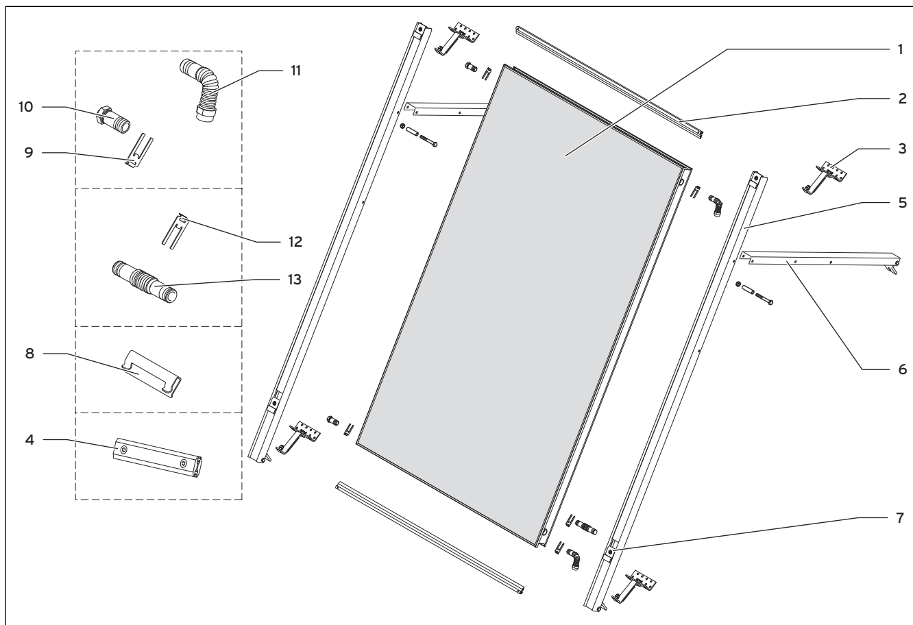
Рис. 5.3 Монтажный комплект VFK 135/2 VD
