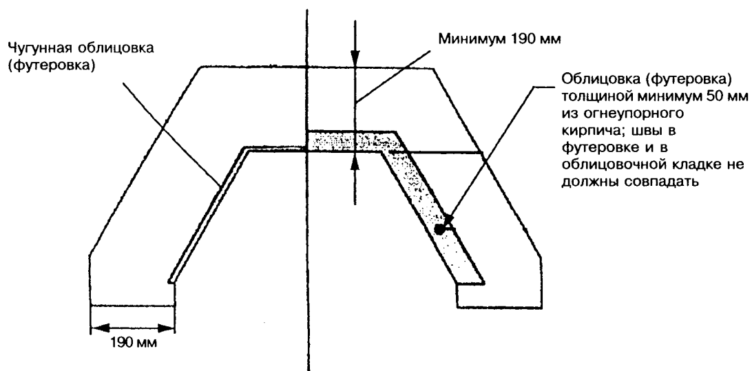
Рисунок 7.5 — Футеровка камина
