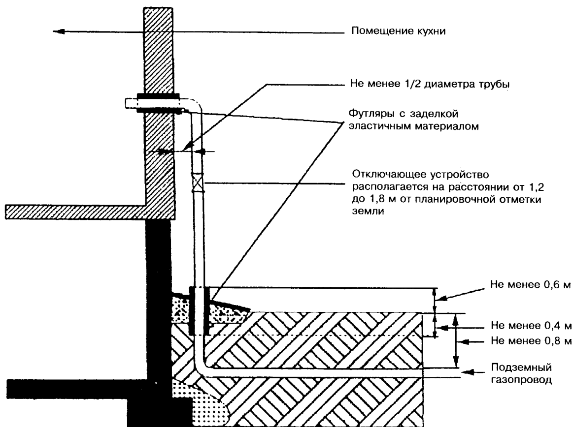
Рисунок 9.1 — Газовый ввод
