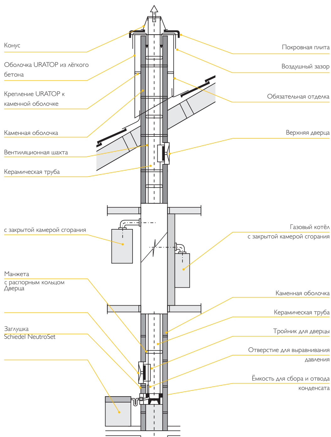
Схема Schiedel Quadro
