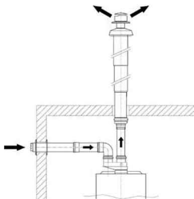
6/11 Раздельное дымоотведение по C52
