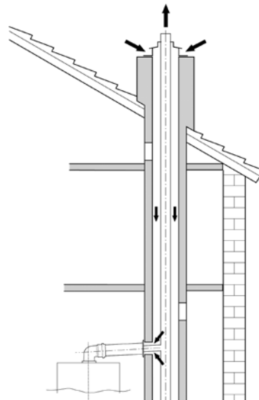
6/10 Концентрическое дымоотведение по C42x
