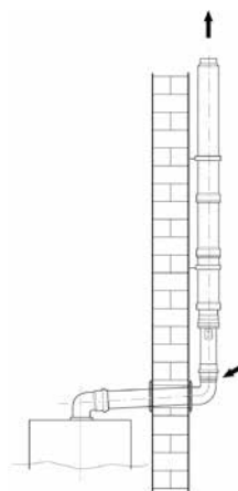
6/12 Концентрическое дымоотведение по C52x
