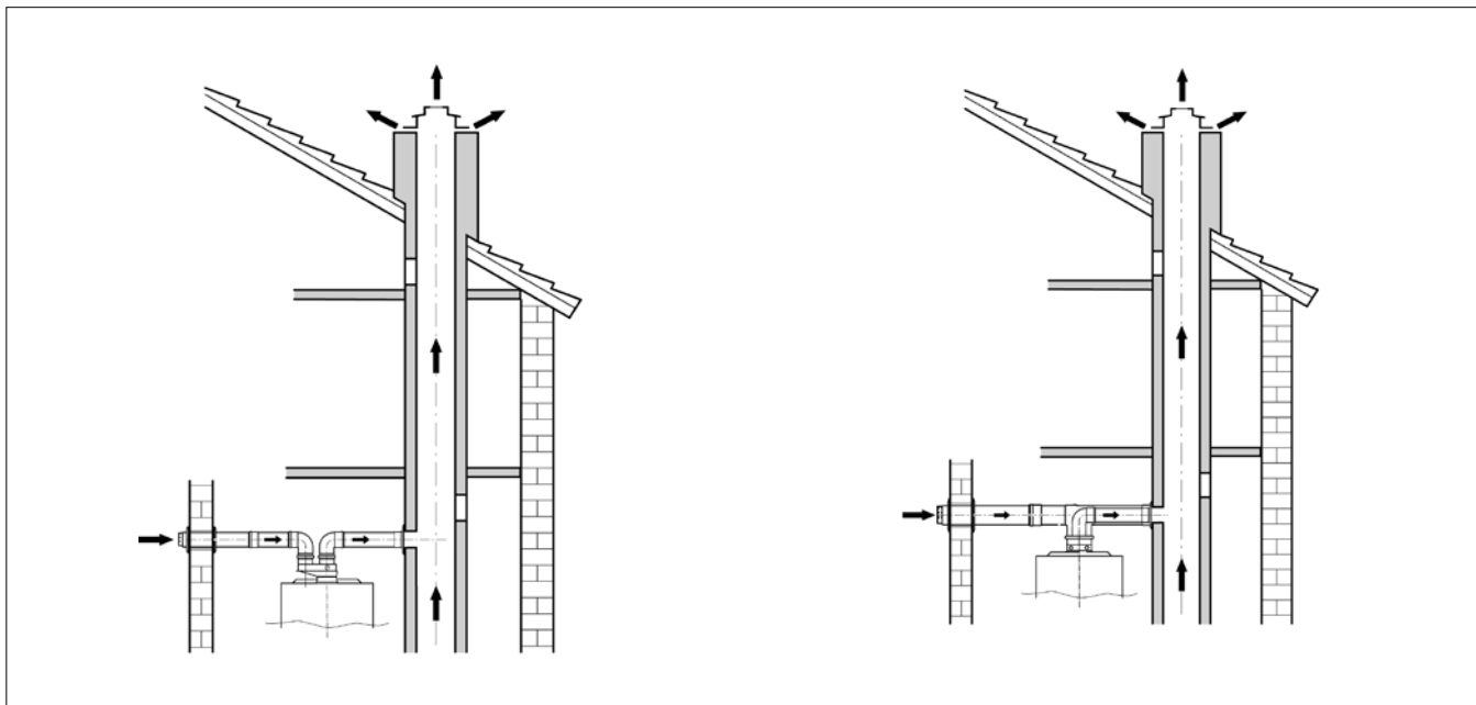
6/13 Раздельное дымоотведение по С82
