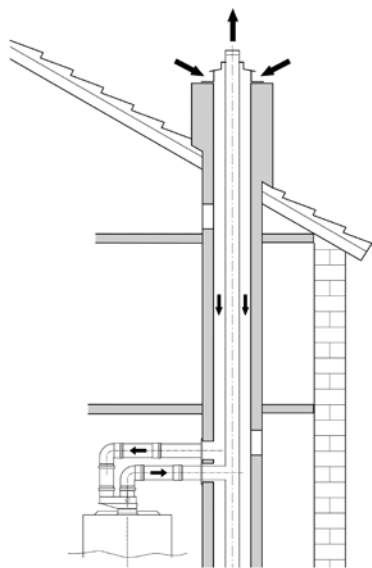
6/9 Раздельное дымоотведение по C42
