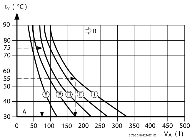
2/2 Диаграмма характеристических кривых расширительного бака котла Logamax U072
