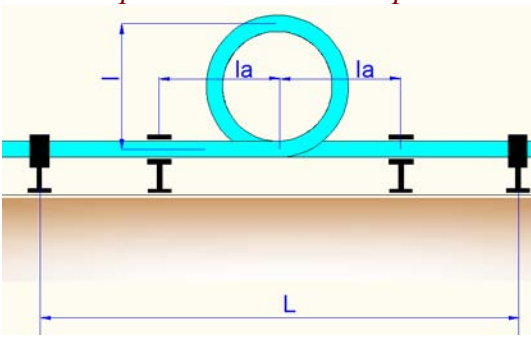
Петлеобразный компенсатор
