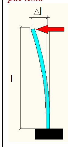
Рис.4.2.4.р.4 Консольная схема расчета
