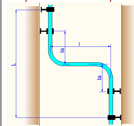
Z-образный компенсатор
