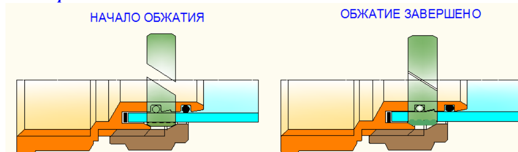
Рис.3.4.р.2. Стадии обжатия МПТ
