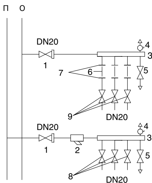
ПРИНЦИПИАЛЬНАЯ СХЕМА
