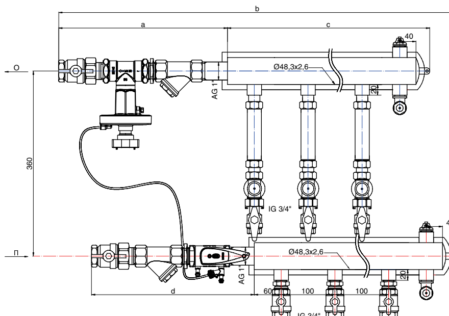
ПРИНЦИПИАЛЬНАЯ СХЕМА
