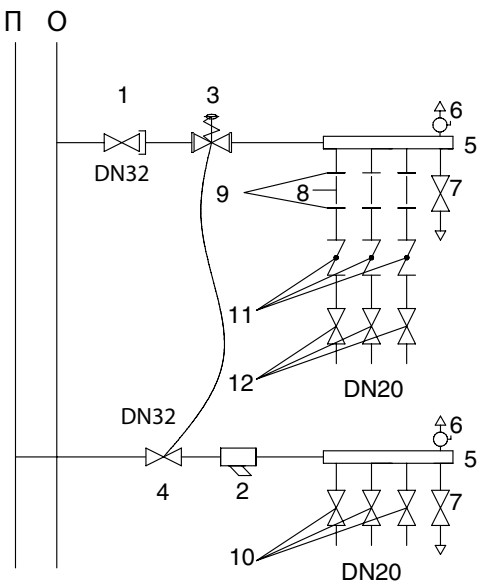
ПРИНЦИПИАЛЬНАЯ СХЕМА
