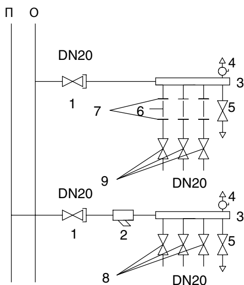
ПРИНЦИПИАЛЬНАЯ СХЕМА
