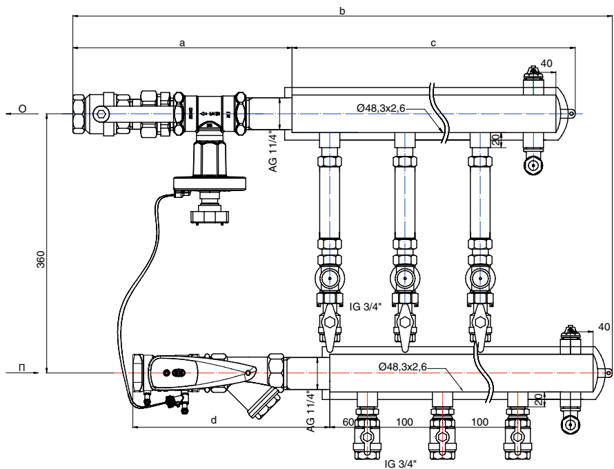
ПРИНЦИПИАЛЬНАЯ СХЕМА
